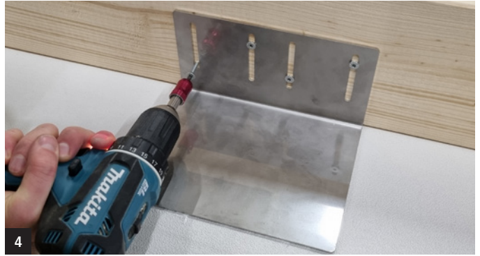
4 Winkel im Riegel verschrauben. Anmerkung: Bei Plattenstößen ist im Bereich des Stoßes ebenfalls ein Winkel vorzusehen
