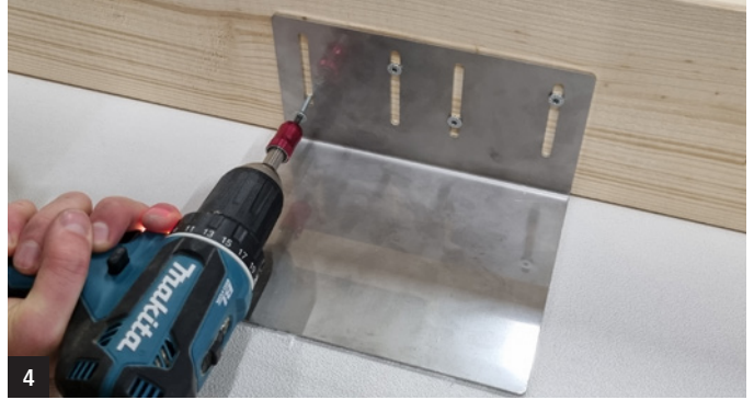
4 Winkel im Riegel verschrauben. Anmerkung: Bei Plattenstößen ist im Bereich des Stosses ebenfalls ein Winkel vorzusehen
