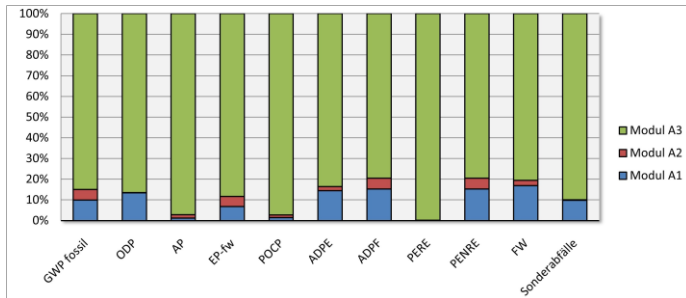
Abb.1: Relative Anteile der Module A1–A3 am Einfluss auf die Umweltwirkungsindikatoren und den Primärenergieeinsatz (cradle-to-gate)
