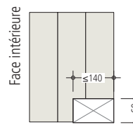
Variante 17 Battue pour semelle de réglage
