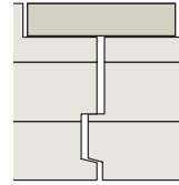
Variante 14 Battue standard 23/51 mm Rainure et languette 10 mm Épaisseur : de 80 mm à 360 mm alternative 28/51 mm Épaisseur : de 90 à 360 mm Battue spéciale max. 39/59 mm
