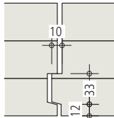
Variante 11 Rainure et languette 10 mm
