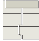
Variante 14 Rainure et crête 10 mm Battue standard 23/51 Épaisseur : de 80 mm à 280 mm Battue spéciale pour 80 mm max. 27/59 à partir de 90 mm max. 35/59
