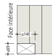
Variante 18 Battue pour semelle de réglage
