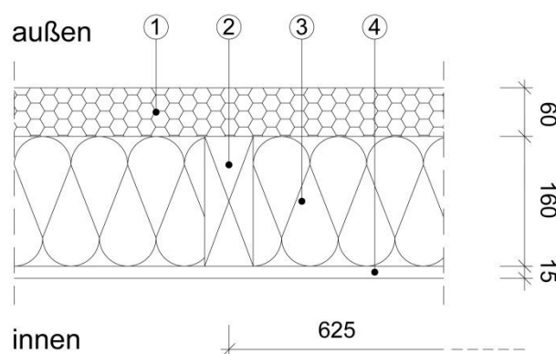
Abbildung 1 Schichtaufbau der Wandkonstruktion
