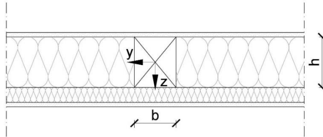
Abbildung 2 Definition der Achsenbezeichnung des Ständers (Beispielbild)
